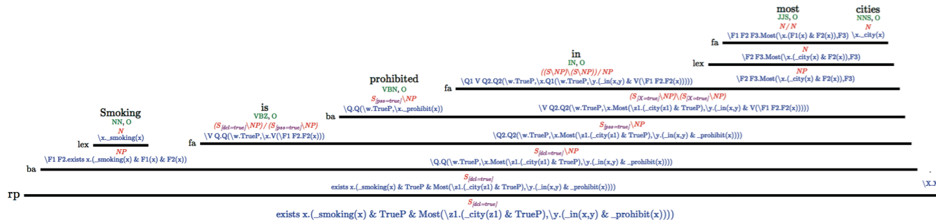
Combinatory Categorical Grammarによる構文・意味解析。文の構造に沿って意味表現を合成し、「Smoking is prohibited in most cities.」という文から「Some cities allow smoking.」が言えるか、といった計算を行う。
