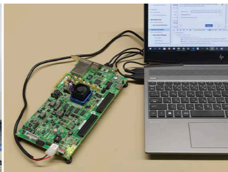
FPGAに論理回路のデータを送り込んでテストする。
